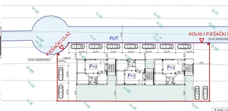
SITUACIJA M 1:200
