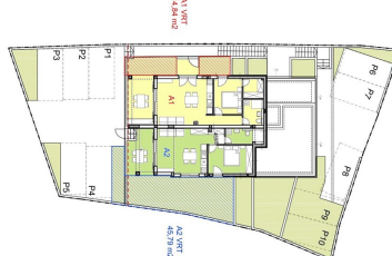
SITUACIA - SUTEREN
