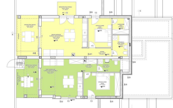
SUTEREN
