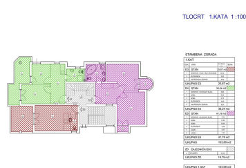
TLOCRT 1.KATA 1:100
