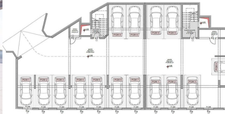
Půdorys suterénu
