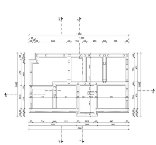
TLOUŠTĚNÉ PŘÍZEMÍ M 1:100
