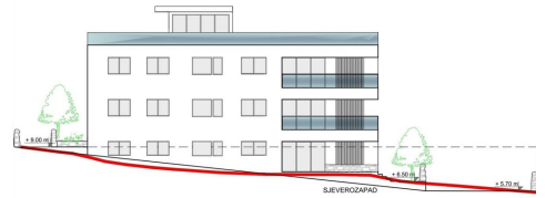
Stambena građevina - KOZINO PRŮČELIA MJ 1:150
