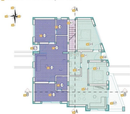
TLOCRT PRIZEMLJA, M 1:100
